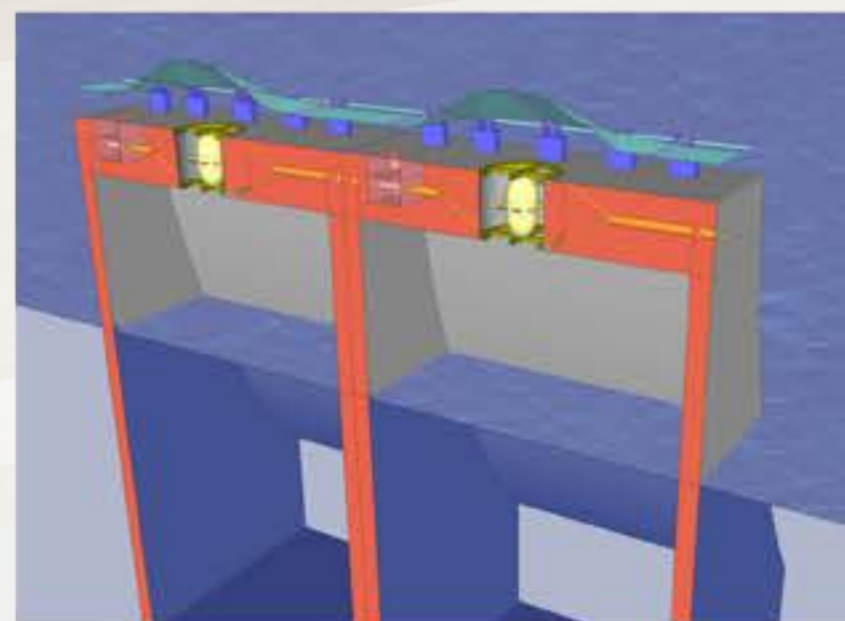
Axonometric Section
