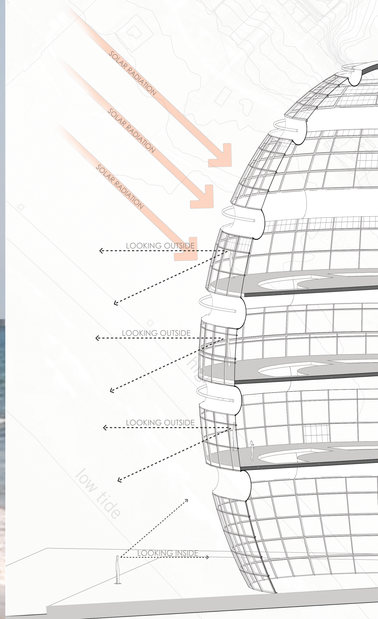
CORSS SECTION
